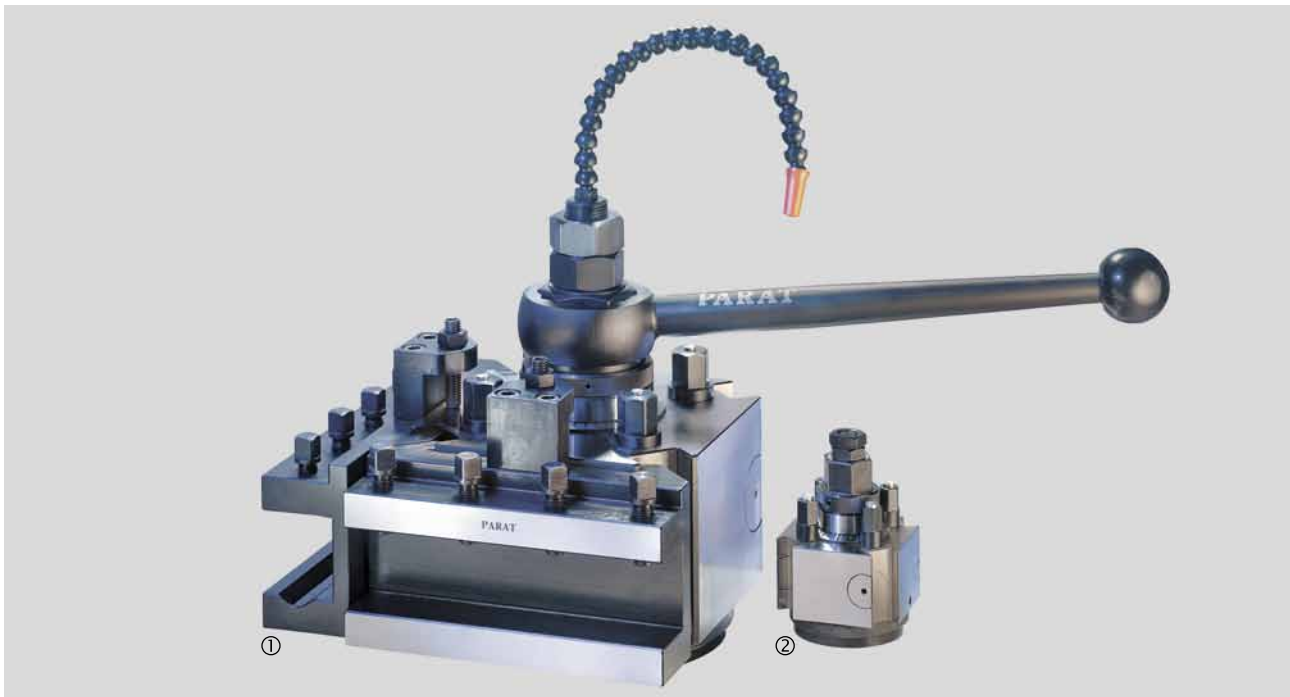
① PARAT-Revolverkopf RD 5
