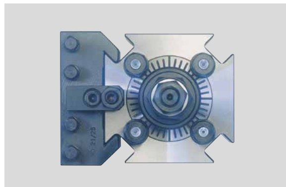
RD 2 mit Wechselhalter WD 2/25
