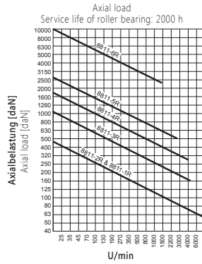
Axialbelastung Lebensdauer des Wälzlagers: 2000 Std.
