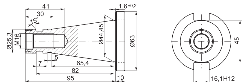
DIN 2080-40
