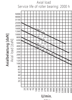
Axialbelastung Lebensdauer des Wälzlagers: 2000 Std.
