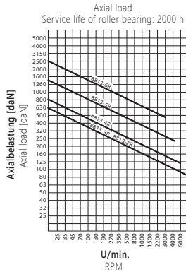
Axialbelastung Lebensdauer des Wälzlagers: 2000 Std.
