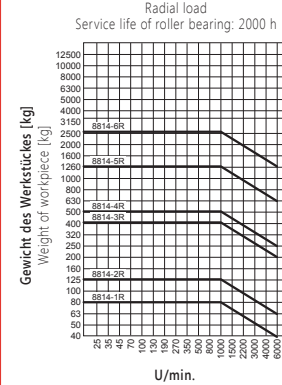
Radialbelastung Lebensdauer des Wälzlagers: 2000 Std.
