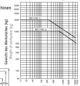
Radialbelastung Lebensdauer des Wälzlagers: 2000 Std. Radial load Service life of roller bearing: 2000 h
