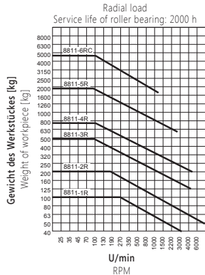
Radialbelastung Lebensdauer des Wälzlagers: 2000 Std.
