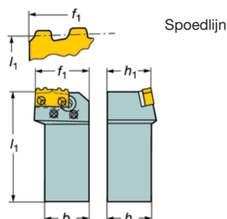
Houder met schacht R166.39FG
