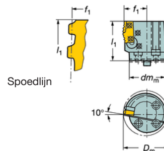
SL snijkop R 566.39KF
